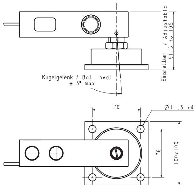
Stoßdämpfer QUICKFIT-S 5t - Damper QUICKFIT-S 5t
