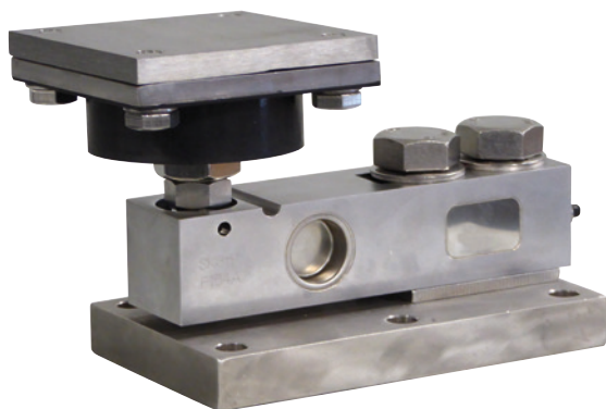
Wägezelle und Stützstange separat erhältlich Load cell and stay rod sold separately
